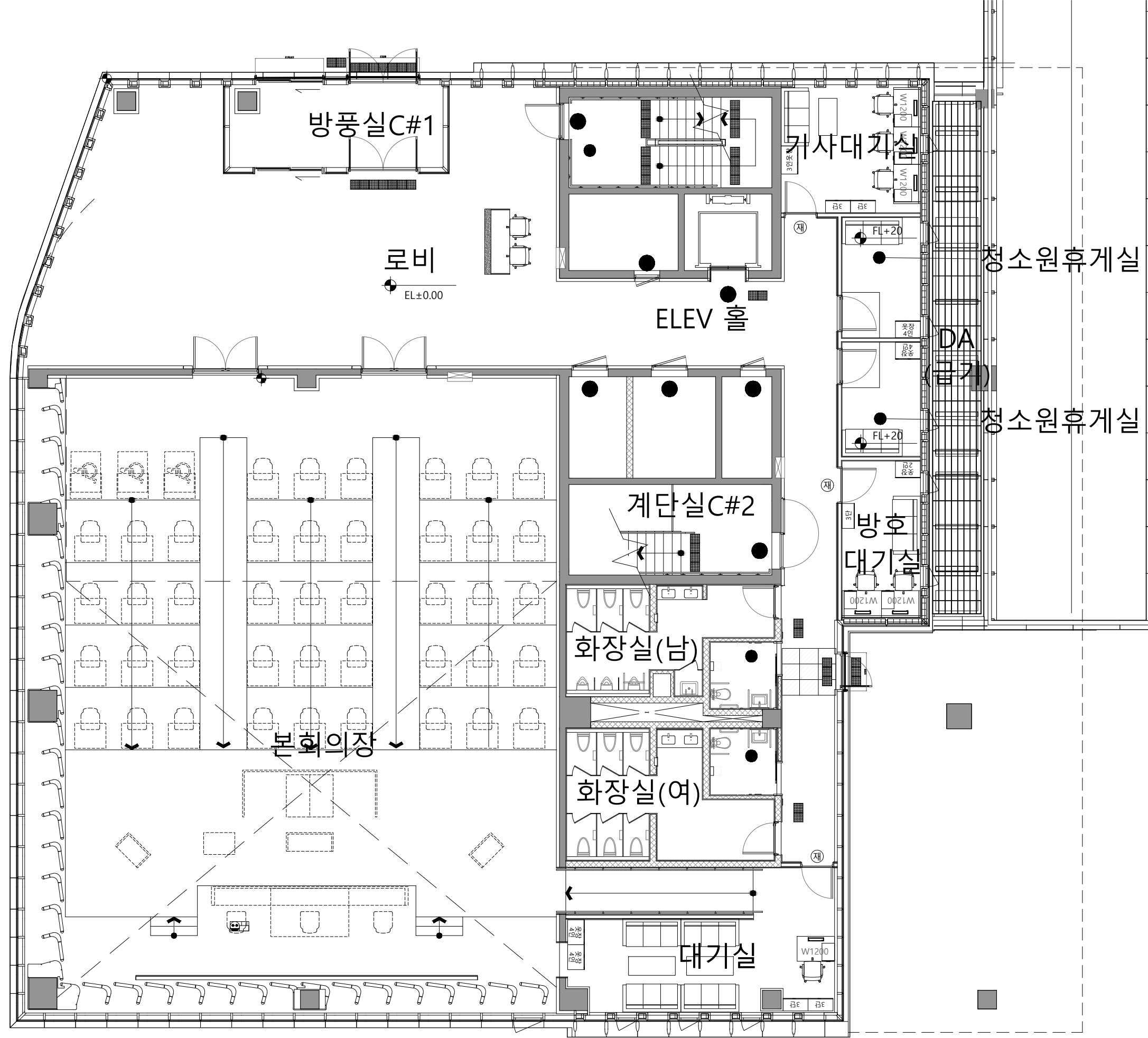
C동(구의회)_1F 평면도
