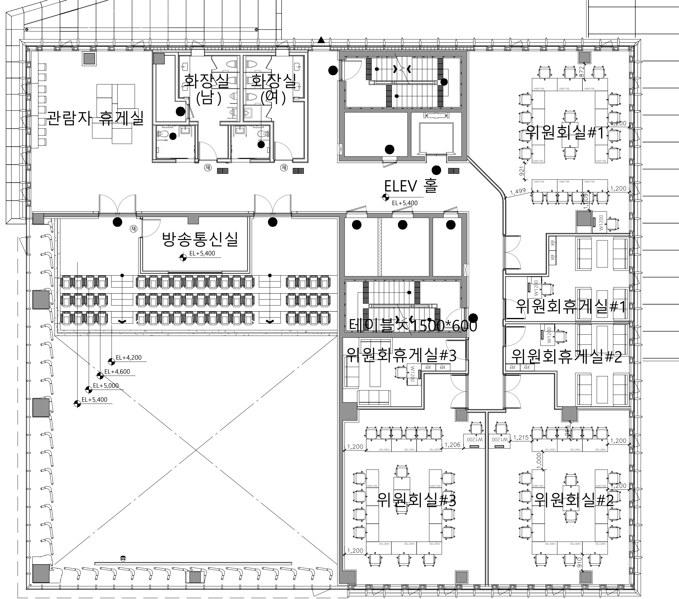
C동(구의회)_2F 평면도
