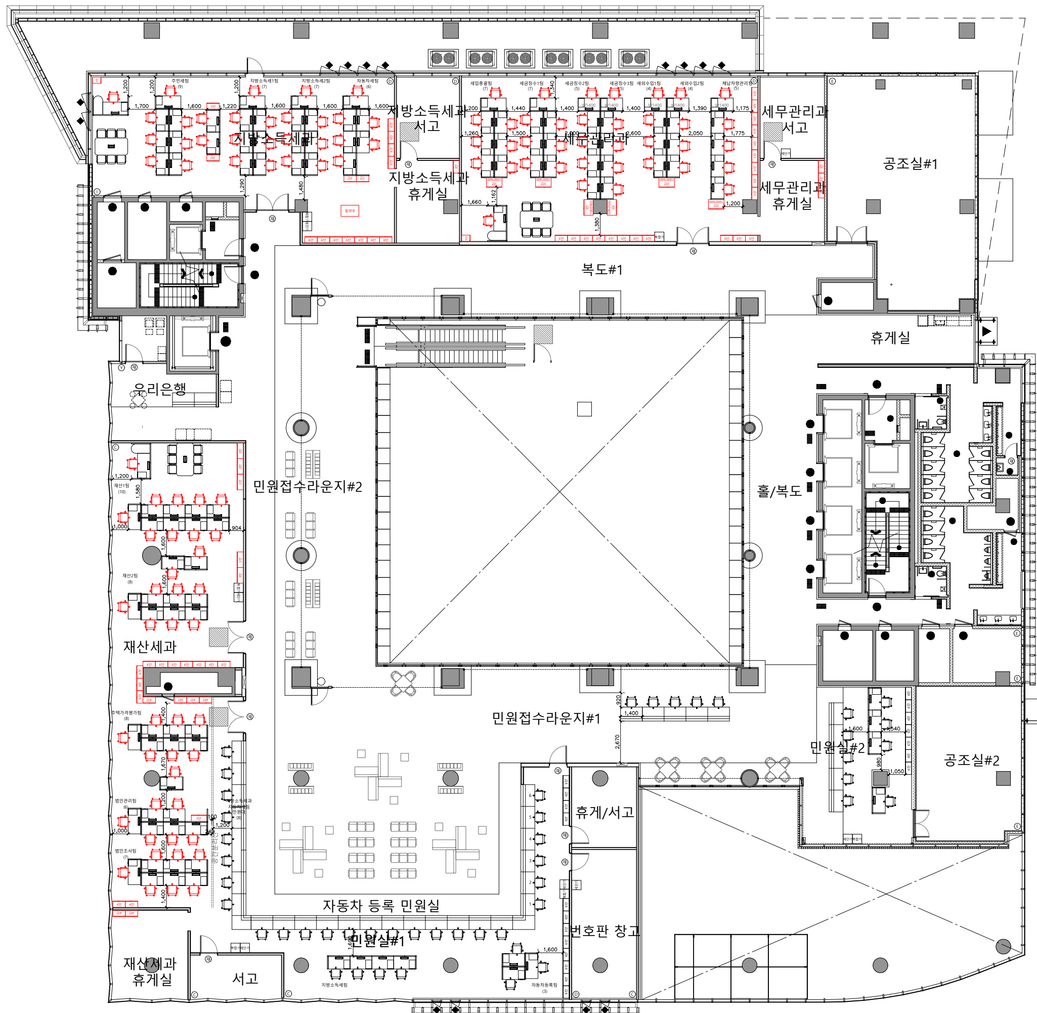
A동(구청사)_2F 평면도
