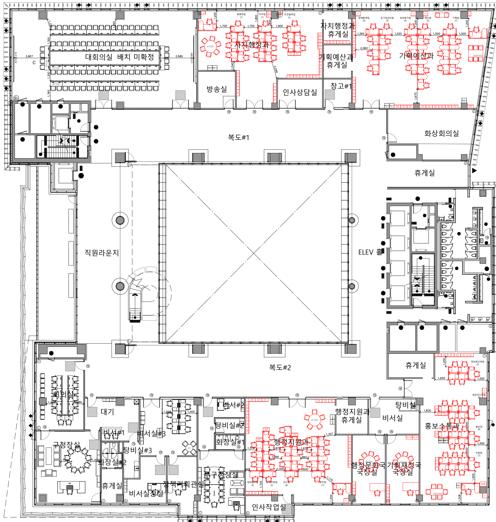
A동(구청사)_3F 평면도
