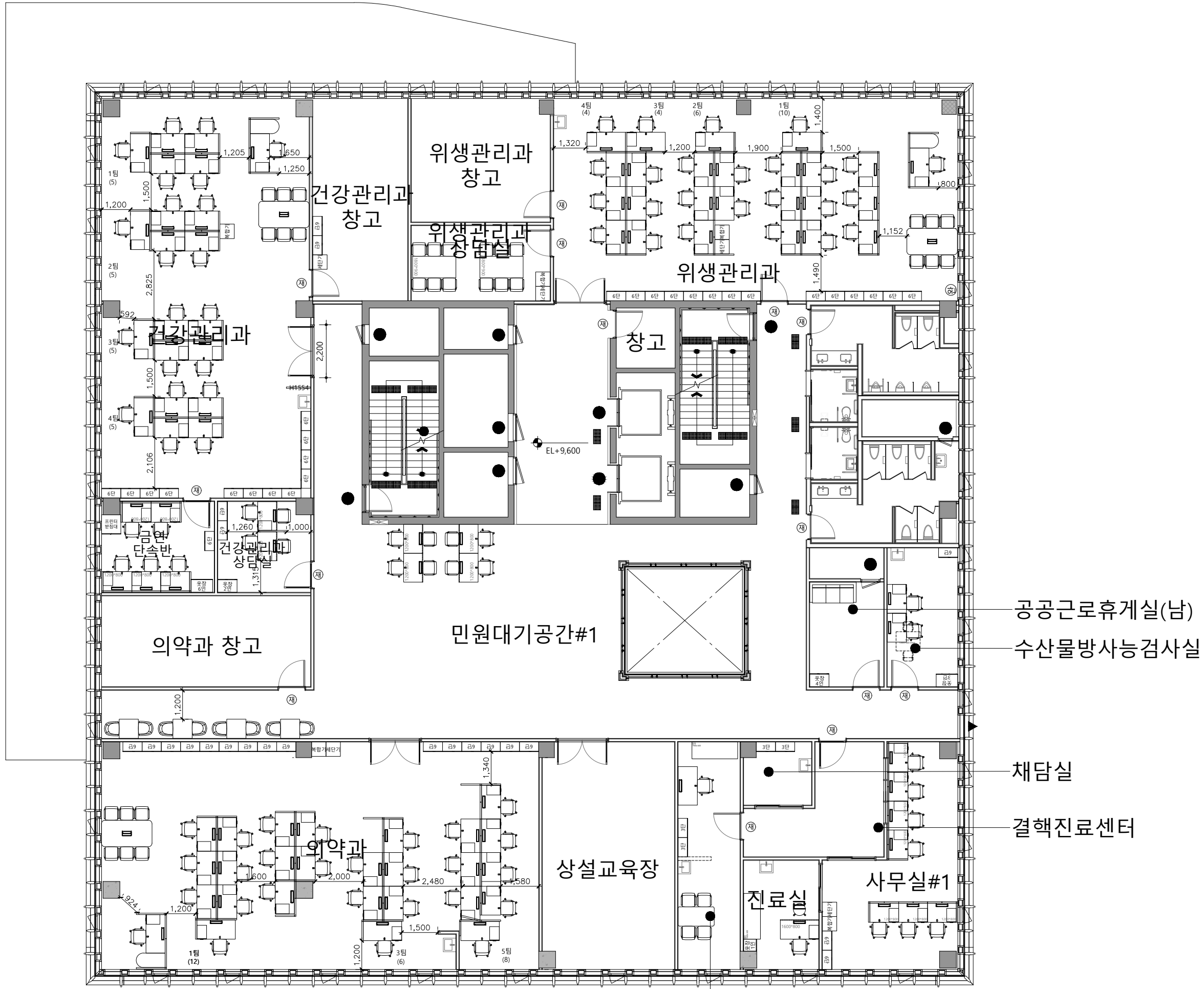
B동(보건소)_3F 평면도
